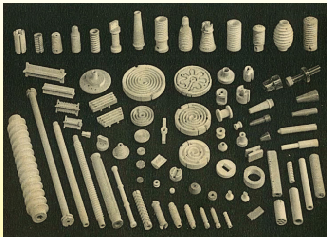
1938年用于电热的滑石绝缘配件 （1938目录书La Stéatite industrielle，Ultimheat博物馆）
