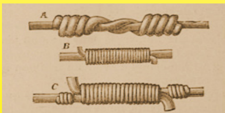
1892年通过绞接电线进行接合（Manuel pratique de l'installation de la lumière électrique. Installations privées, par J.-P. Anney提供的）
